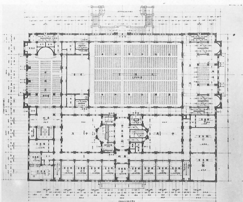
31 東京市政調查會館設計圖選外 O號平面圖
