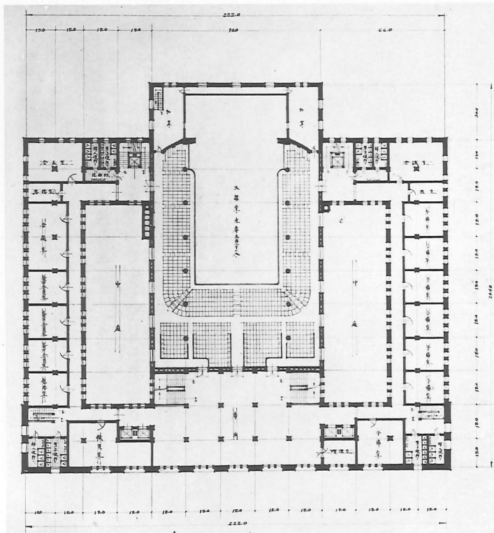
第一階平面圖
