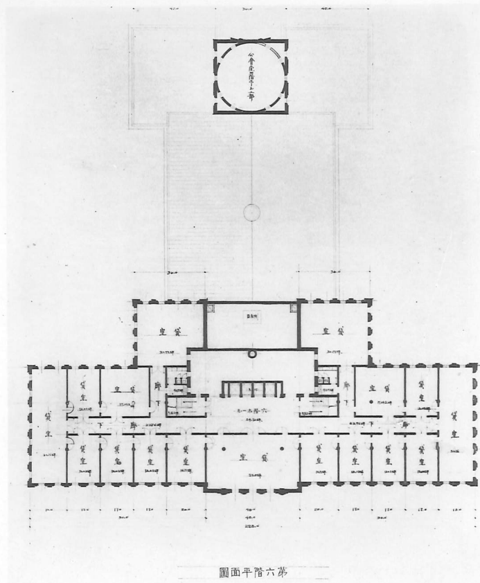
8 東京市政調査會館設計圖一等當選 平面圖 工學博士 佐藤功一氏案
