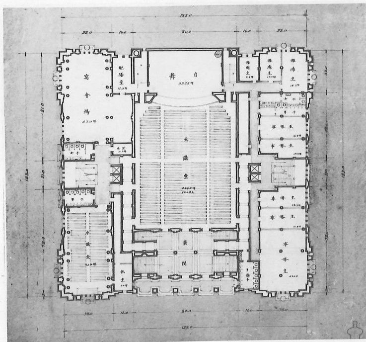
43 東京市政調査會館設計圖選外 I號平面圖
