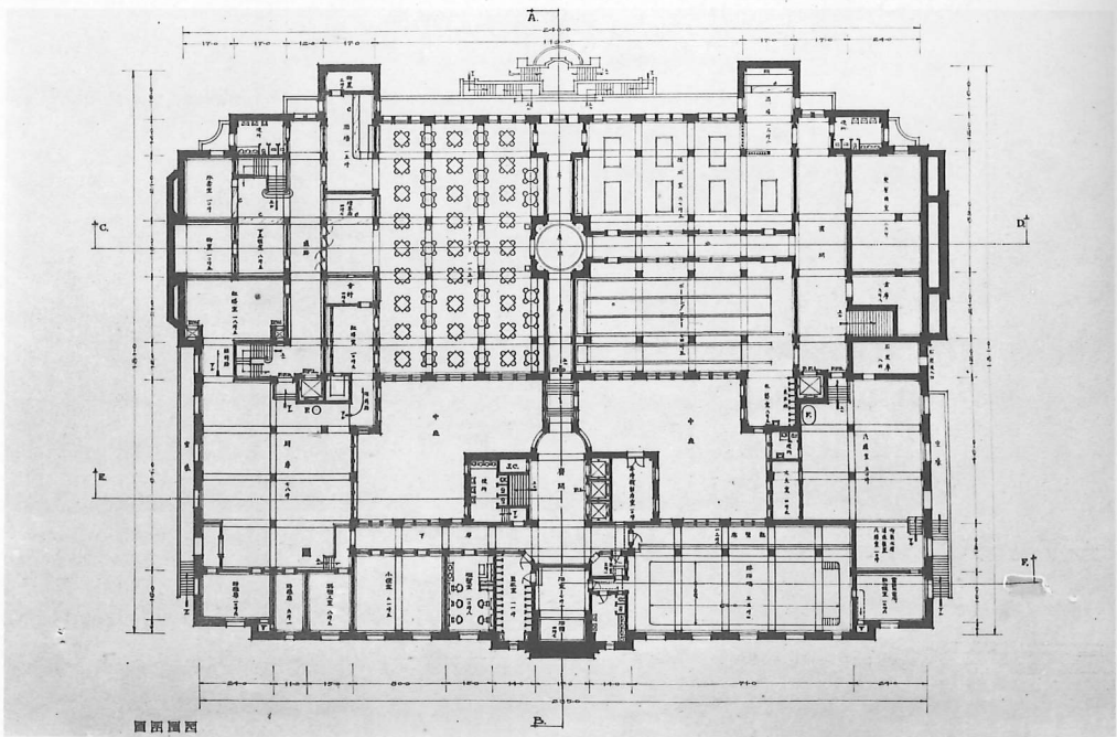
22 東京市政調査會館設計圖三等當選 配置及平面圖 工學士 中條精一郎氏案
