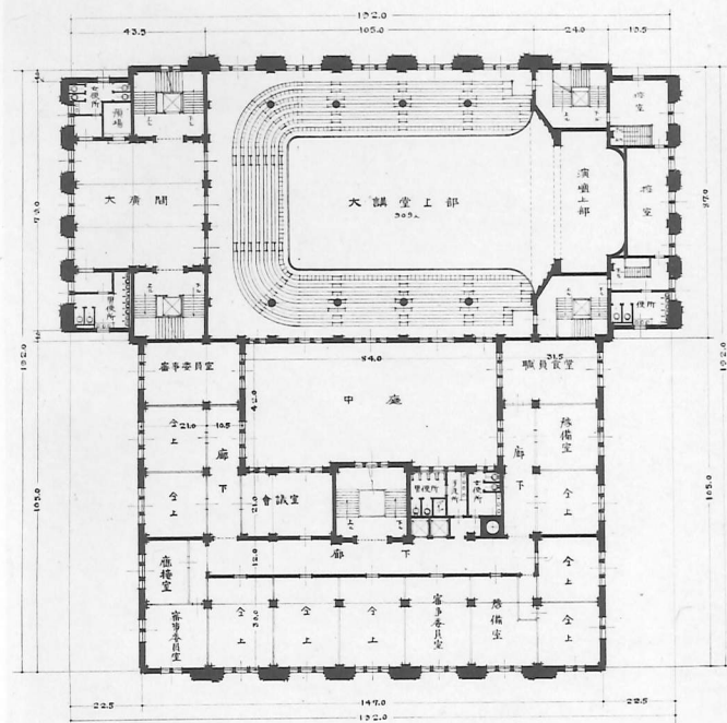
第二階平面圖
