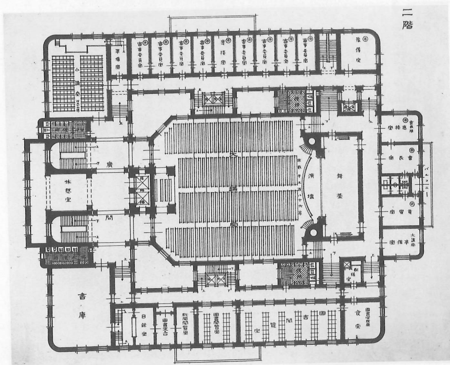
51 東京市政調査會館設計圖選外 M號平面圖
