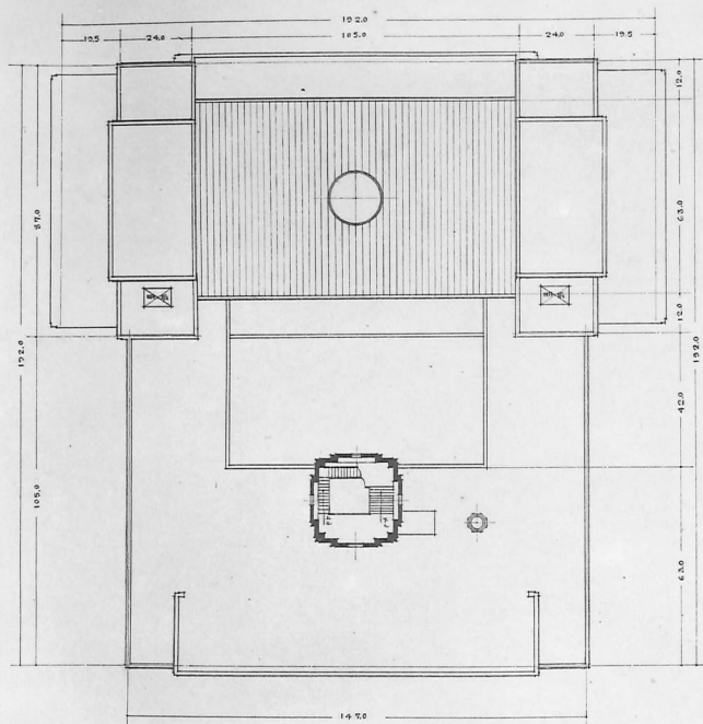
第一層平面圖
