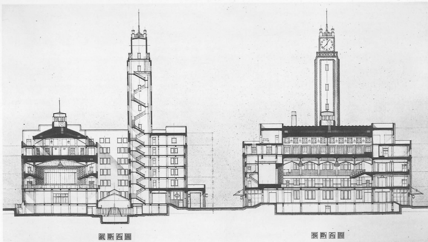
13 東京市政調査會館設計圖二等當選 断面圖 工學士 田邊淳吉氏案
