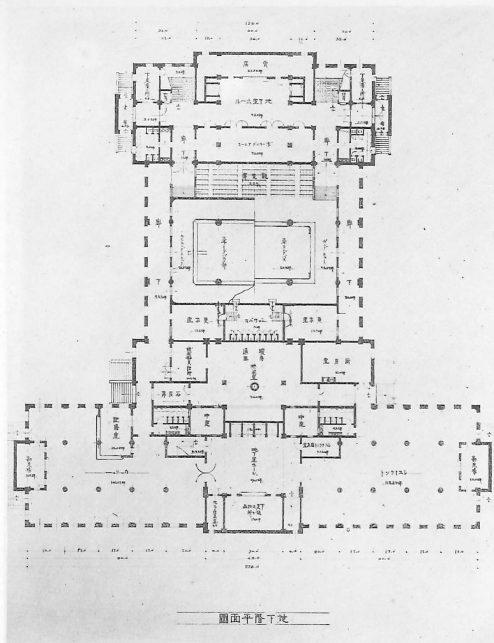
5 東京市政調査会館設計圖一等當選 配置及平面圖 工學博士 佐藤功一氏案
