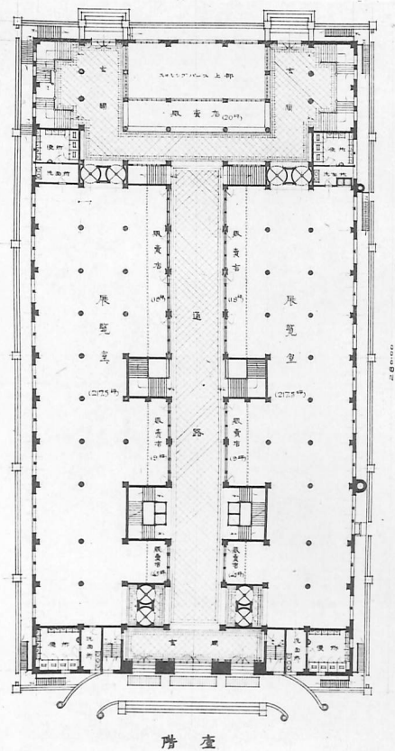
41 東京市政調査會館設計圖選外 II號平面圖
