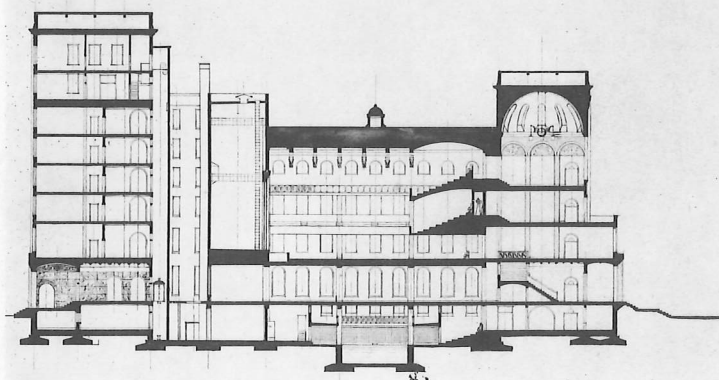
圖面附設會公廳會
