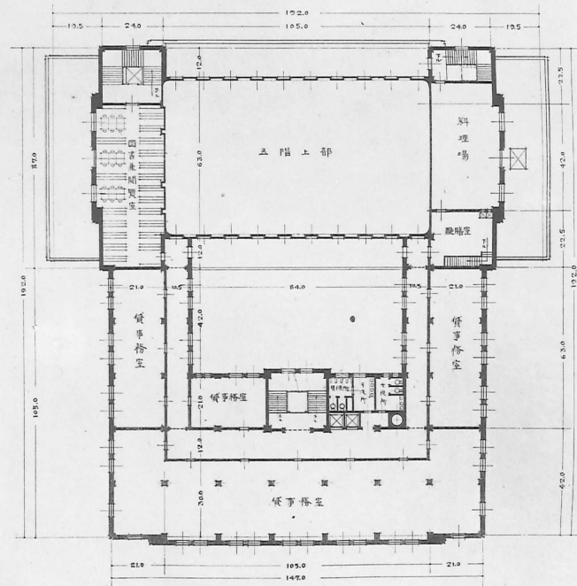
第二層平面圖
