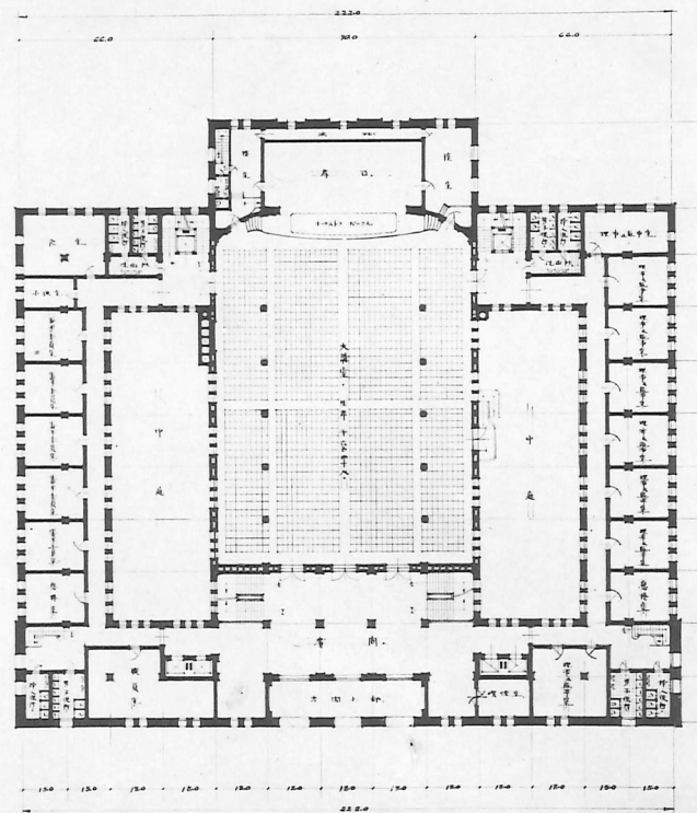
第二階平面圖
