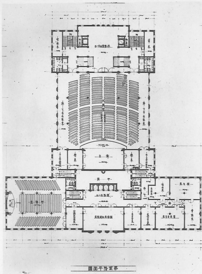
6 東京市政調査會館設計圖一等常選 平面圖 工學博士 佐藤功一氏案
