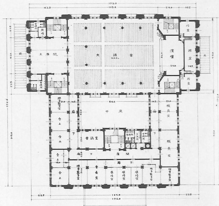
第三階平面圖
