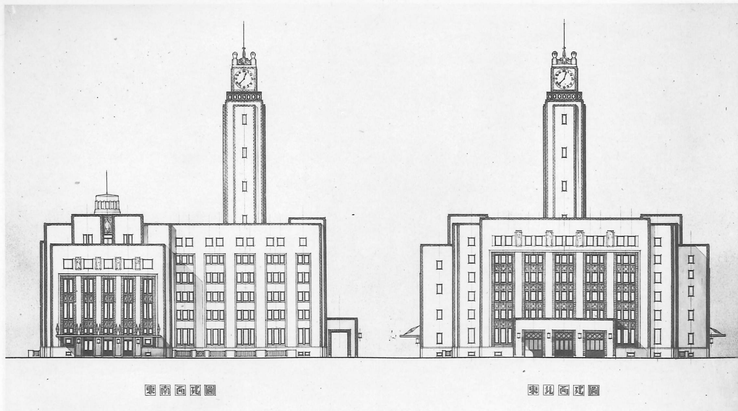
11 東京市政調查會館設計圖二等當選 建圖 工學士 田邊淳吉氏案
