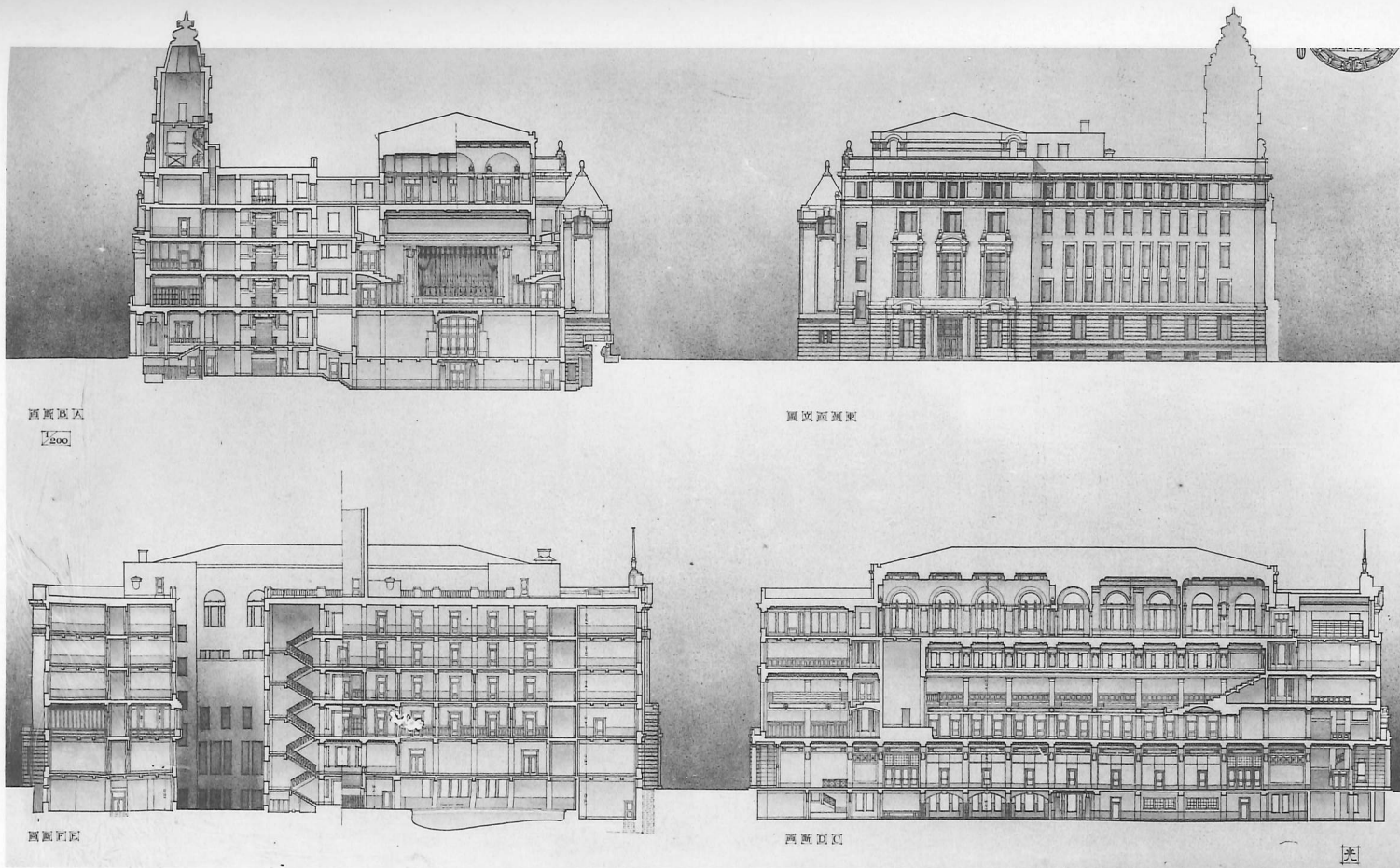
21 東京市政調查會館設計圖三等當選 断面圖 工學士 中條精一郎氏案
